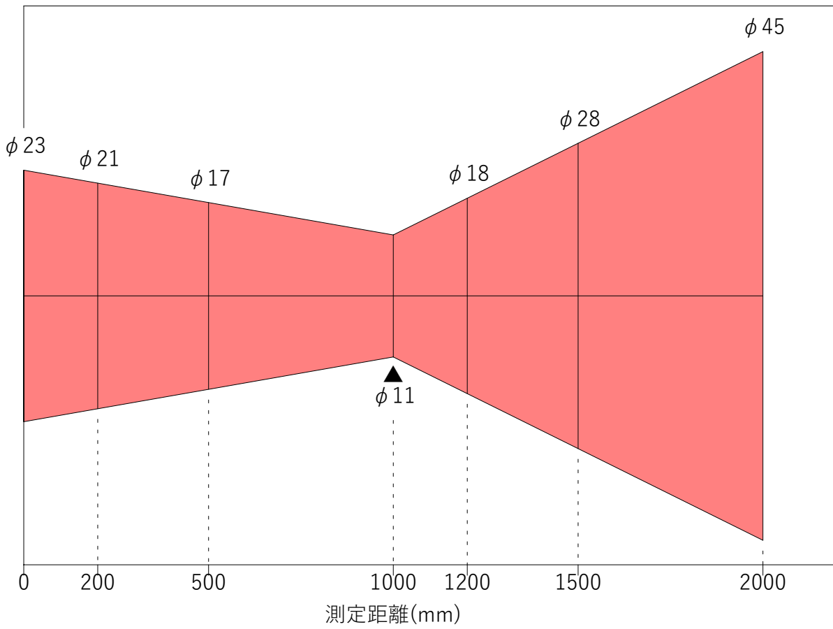
1000H6 光路図
