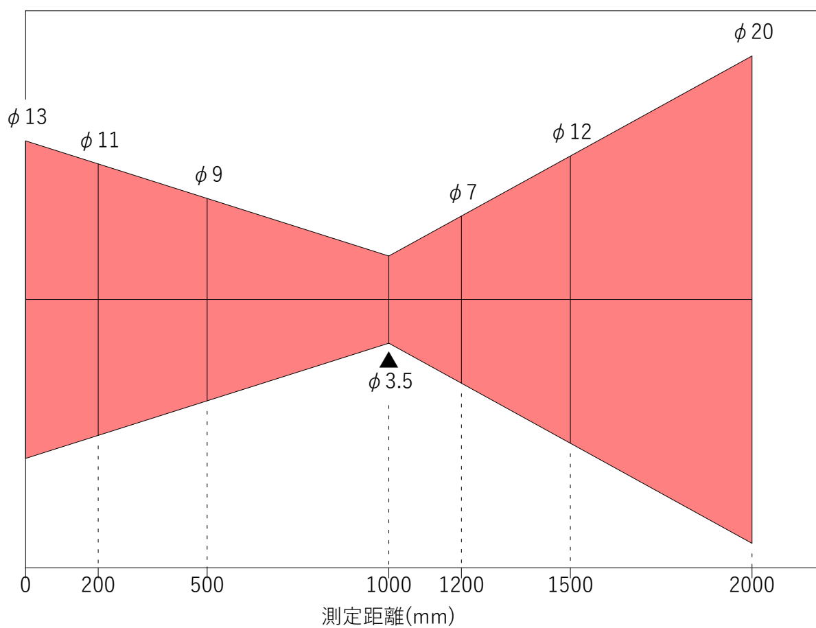
1000B3.5 光路図
