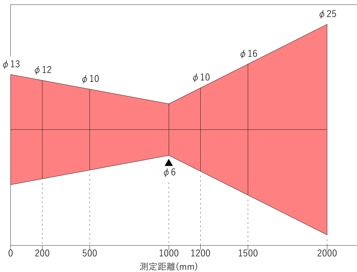
1000B2 光路図
