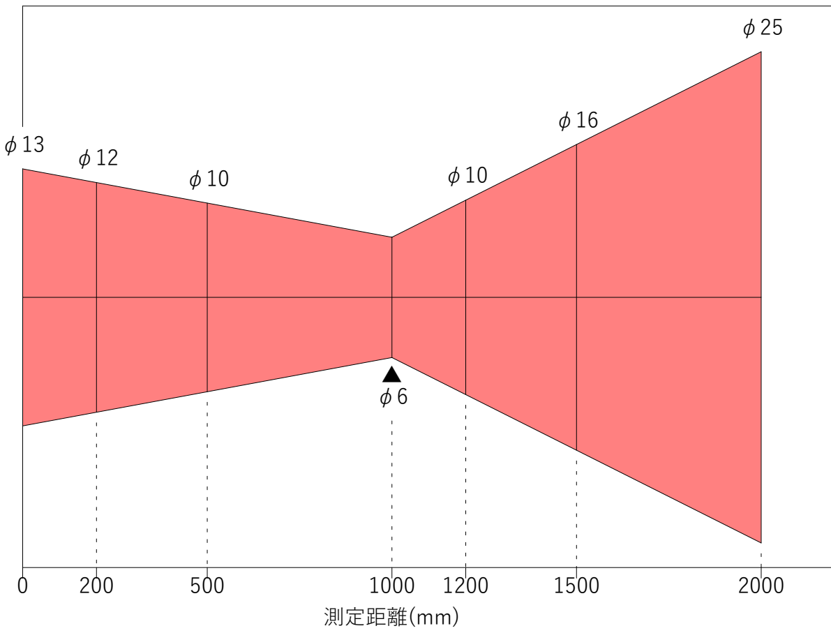
1000B006 光路図
