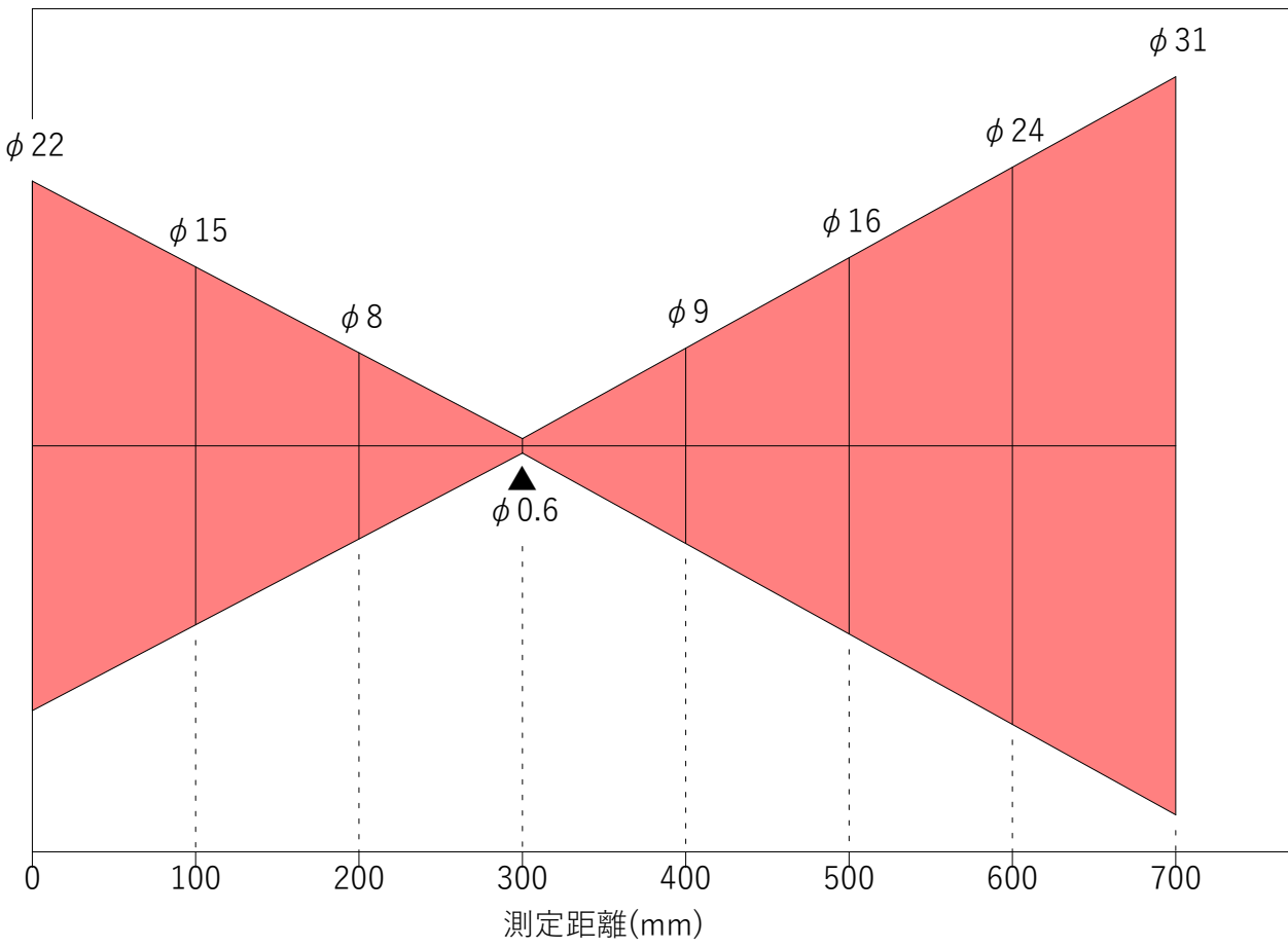
0300H1 光路図
