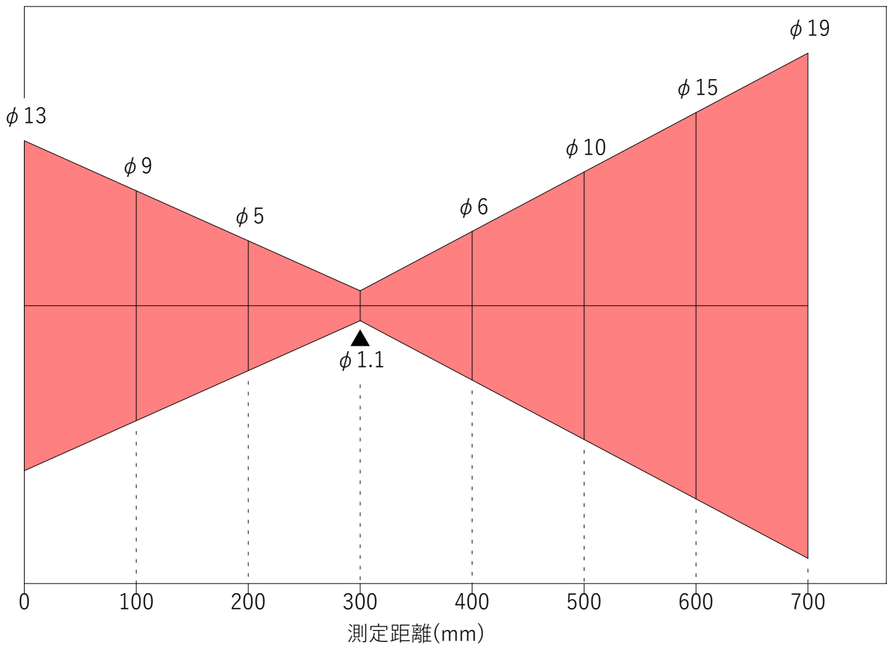
0300B1.1 光路図
