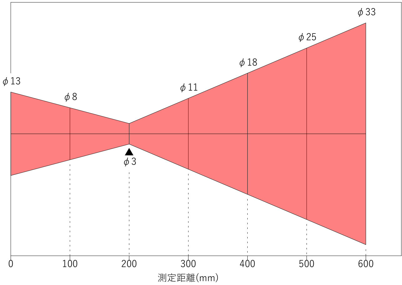
0200B6 光路図
