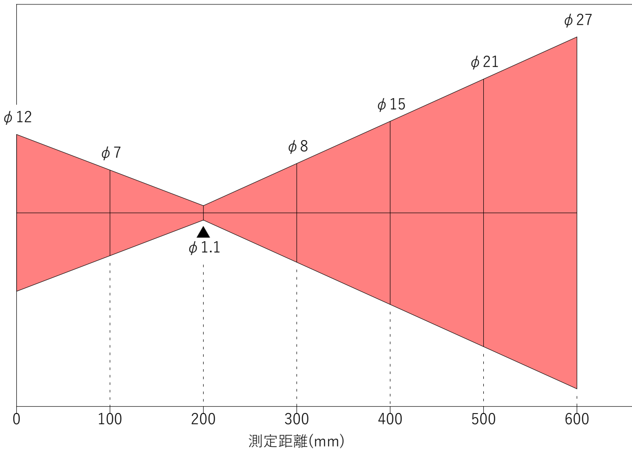
0200B2 光路図
