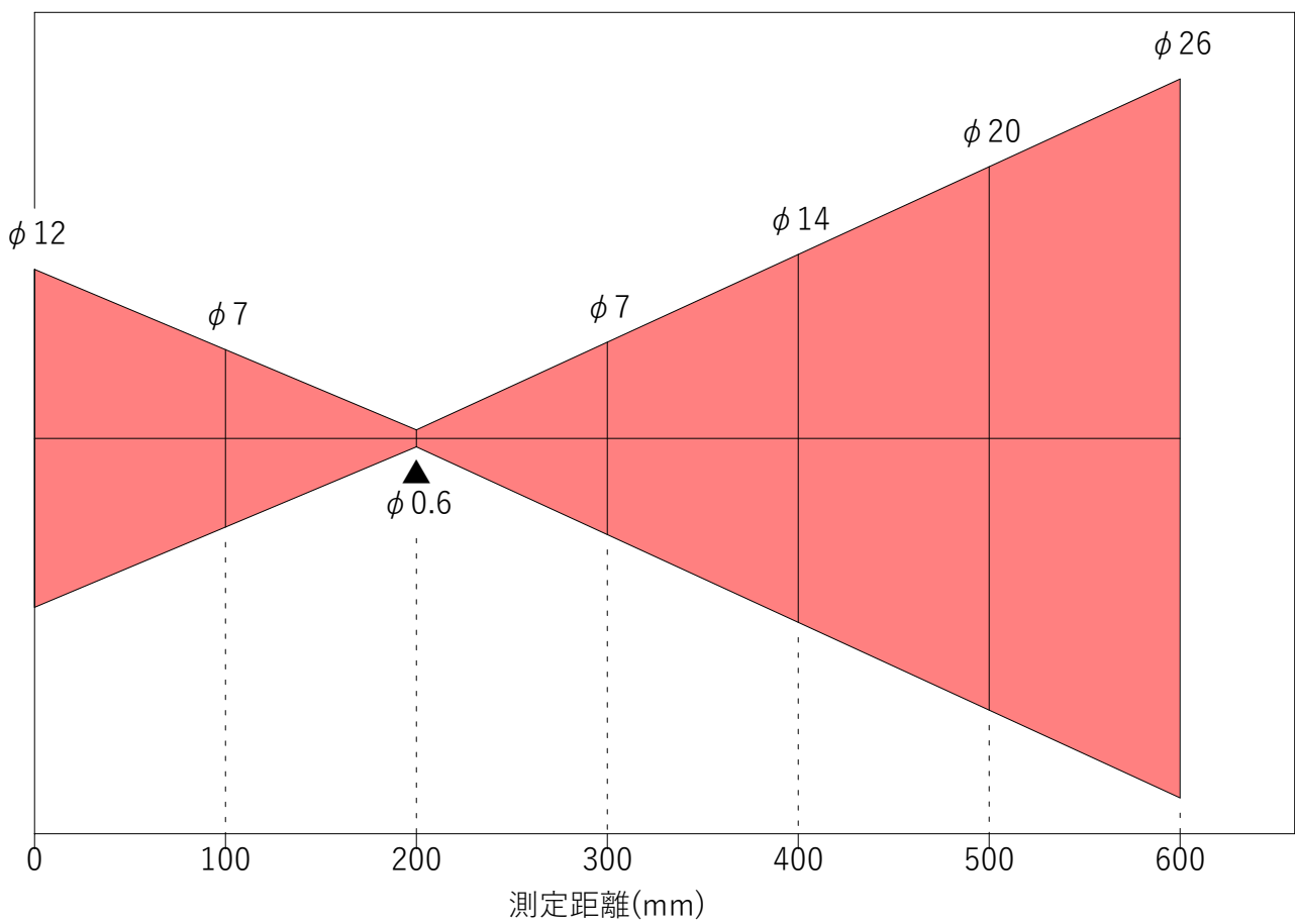
0200B1 光路図
