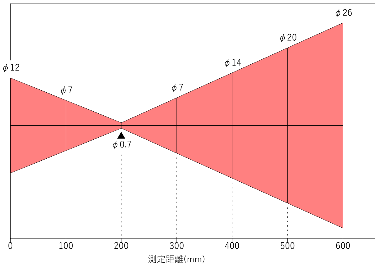
0200B0.7 光路図
