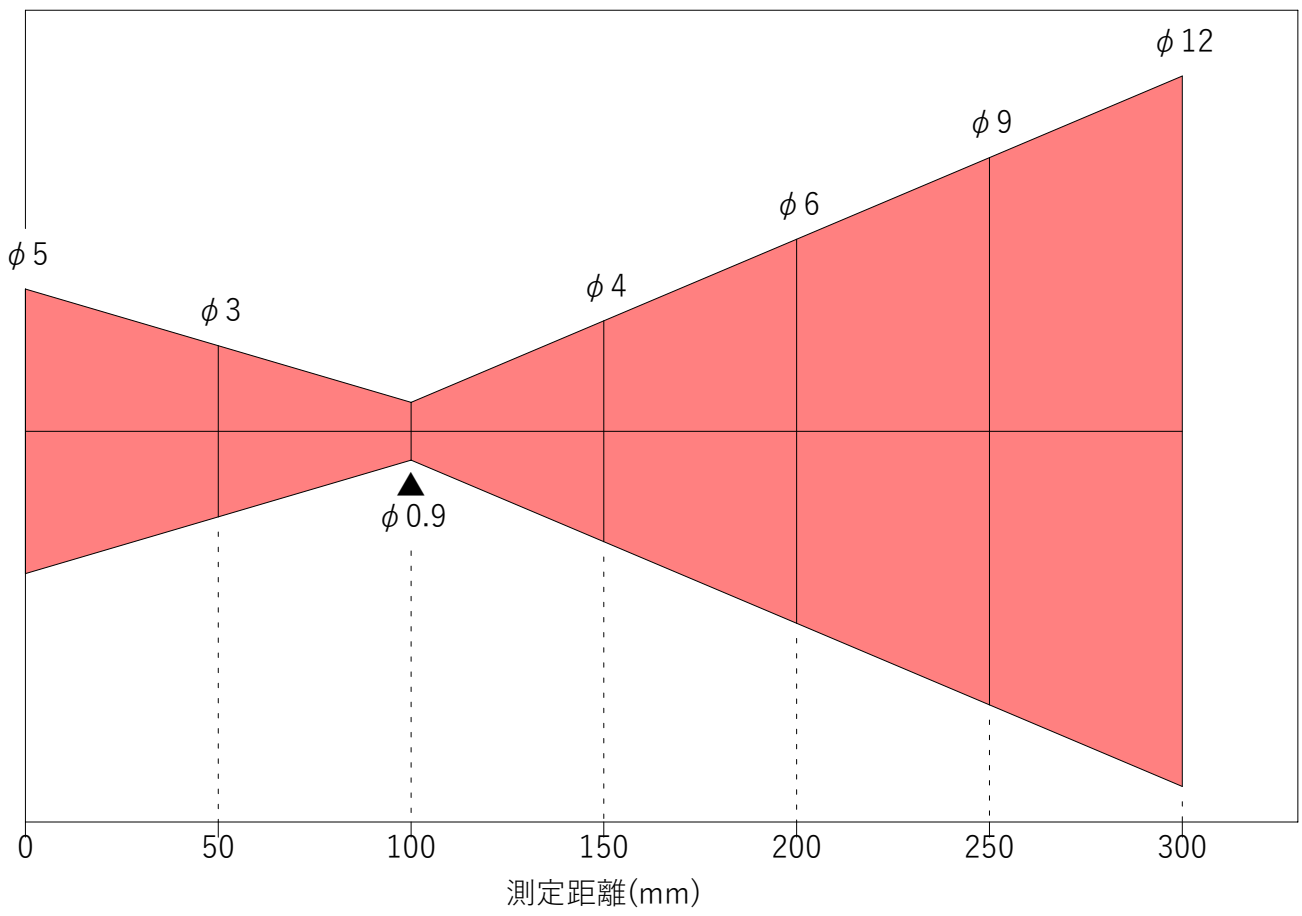
0100S0.9 光路図
