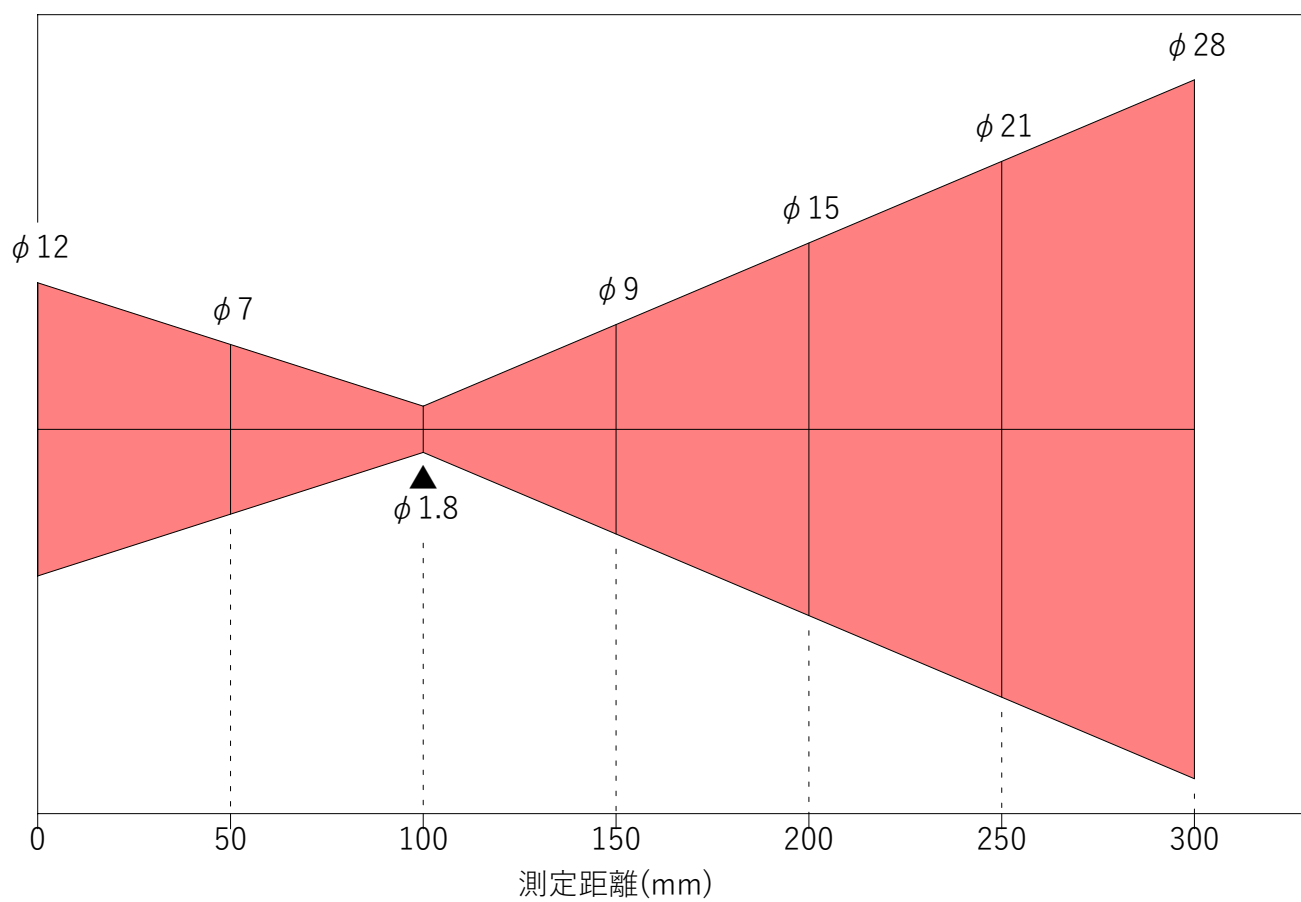
0100B6 光路図
