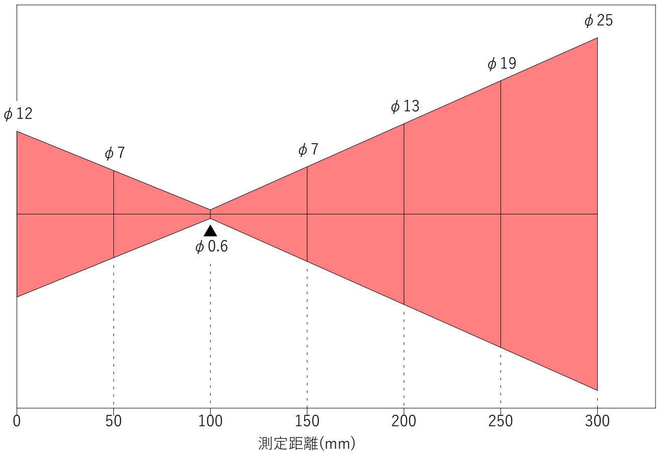
0100B2 光路図
