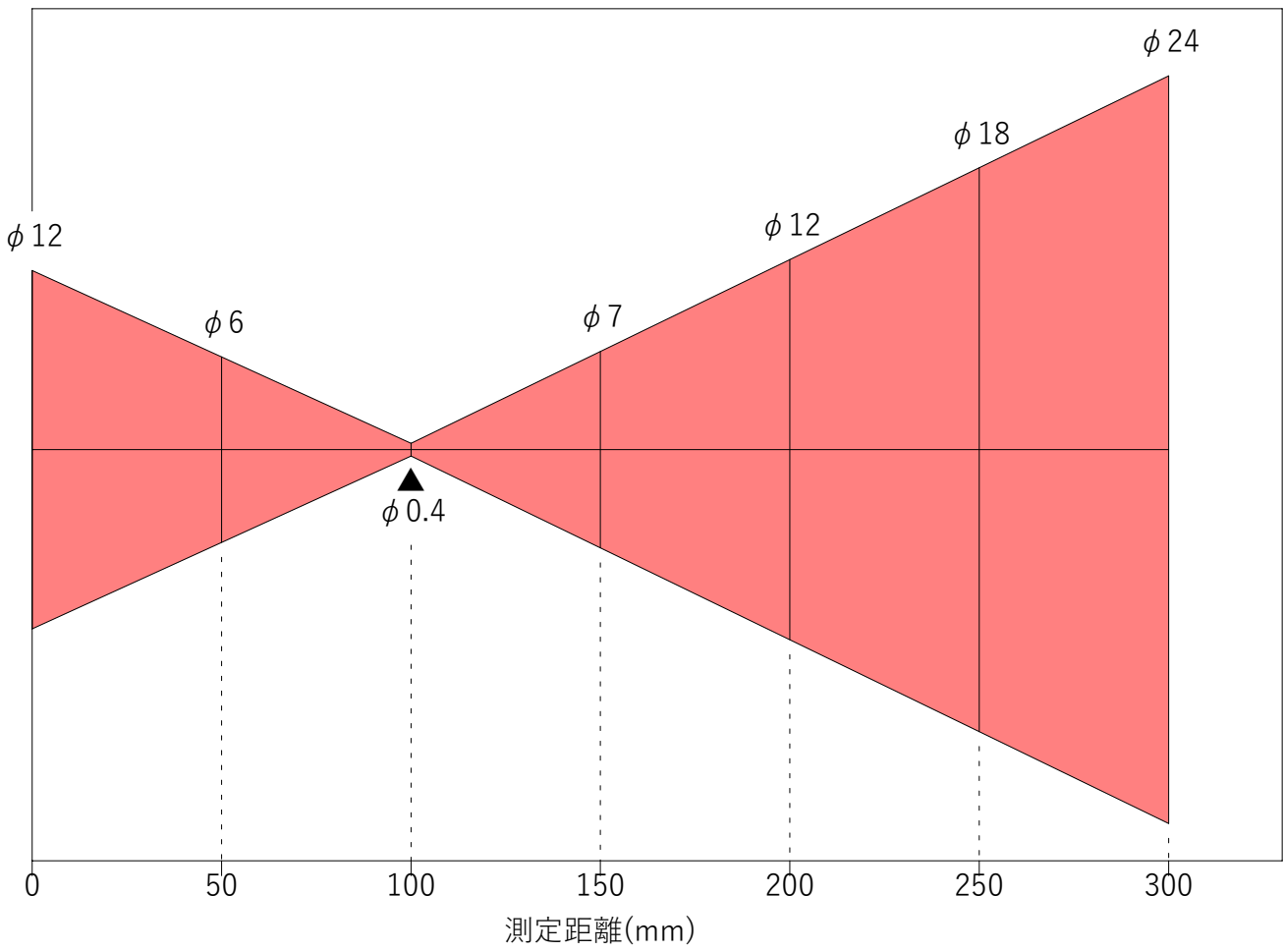
0100B1 光路図
