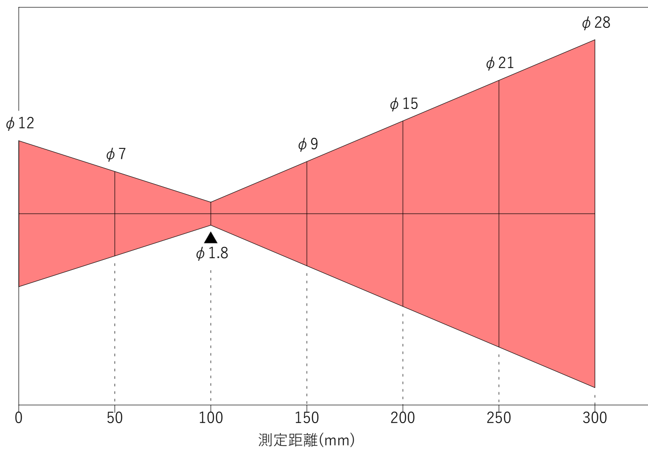
0100B1.8 光路図
