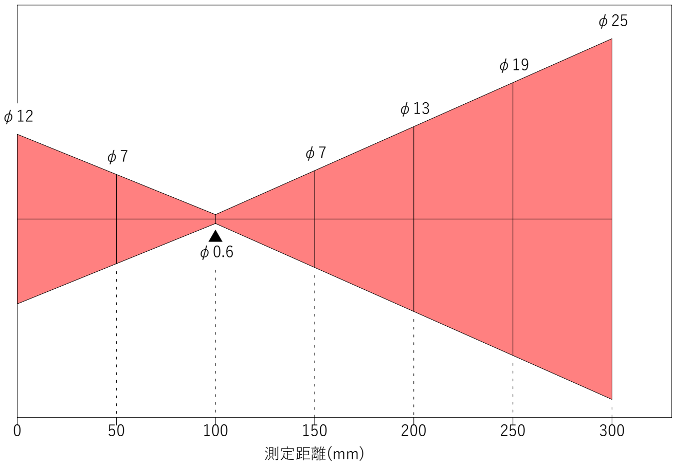
0100B0.6 光路図
