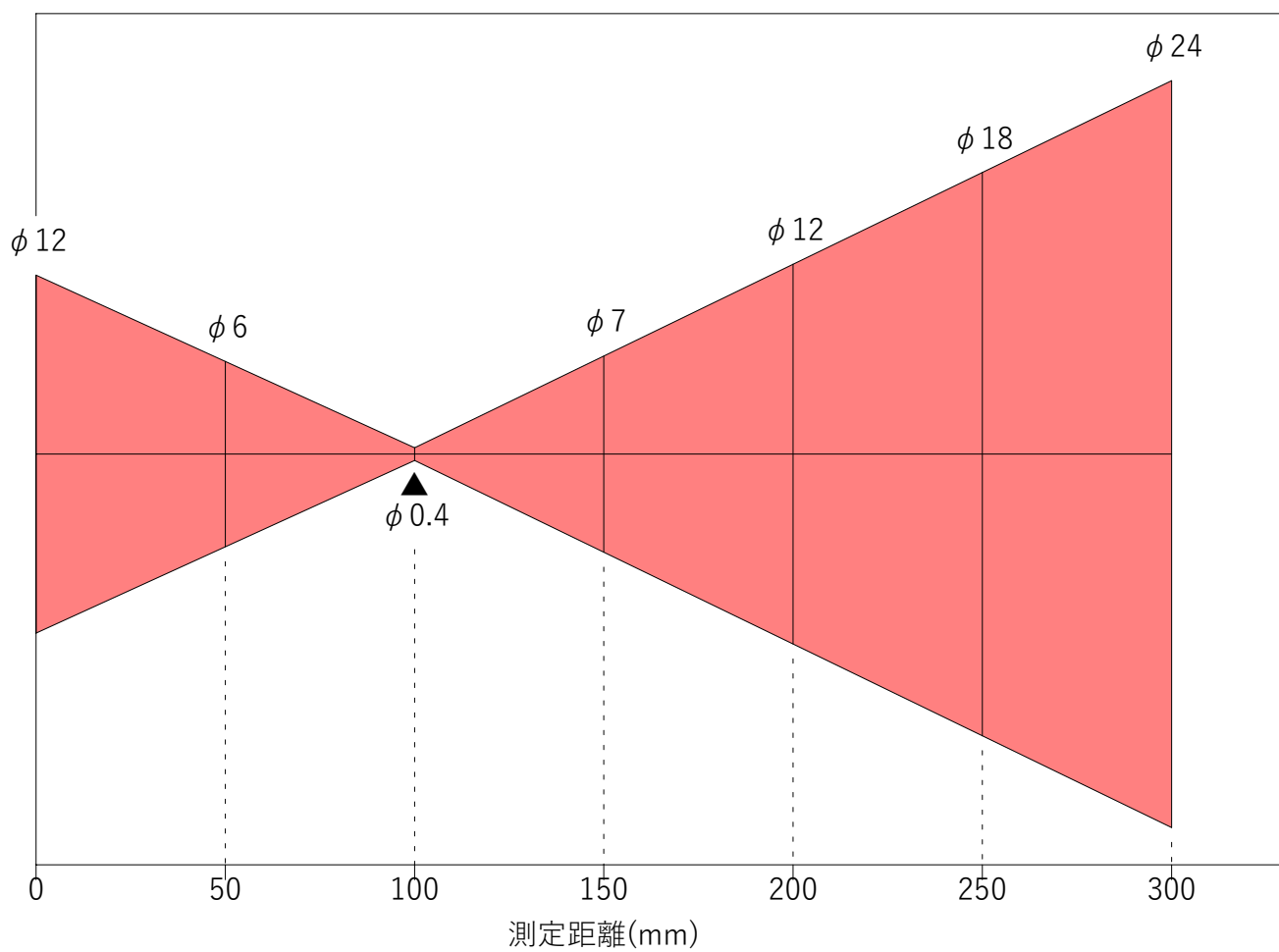
0100B0.4 光路図
