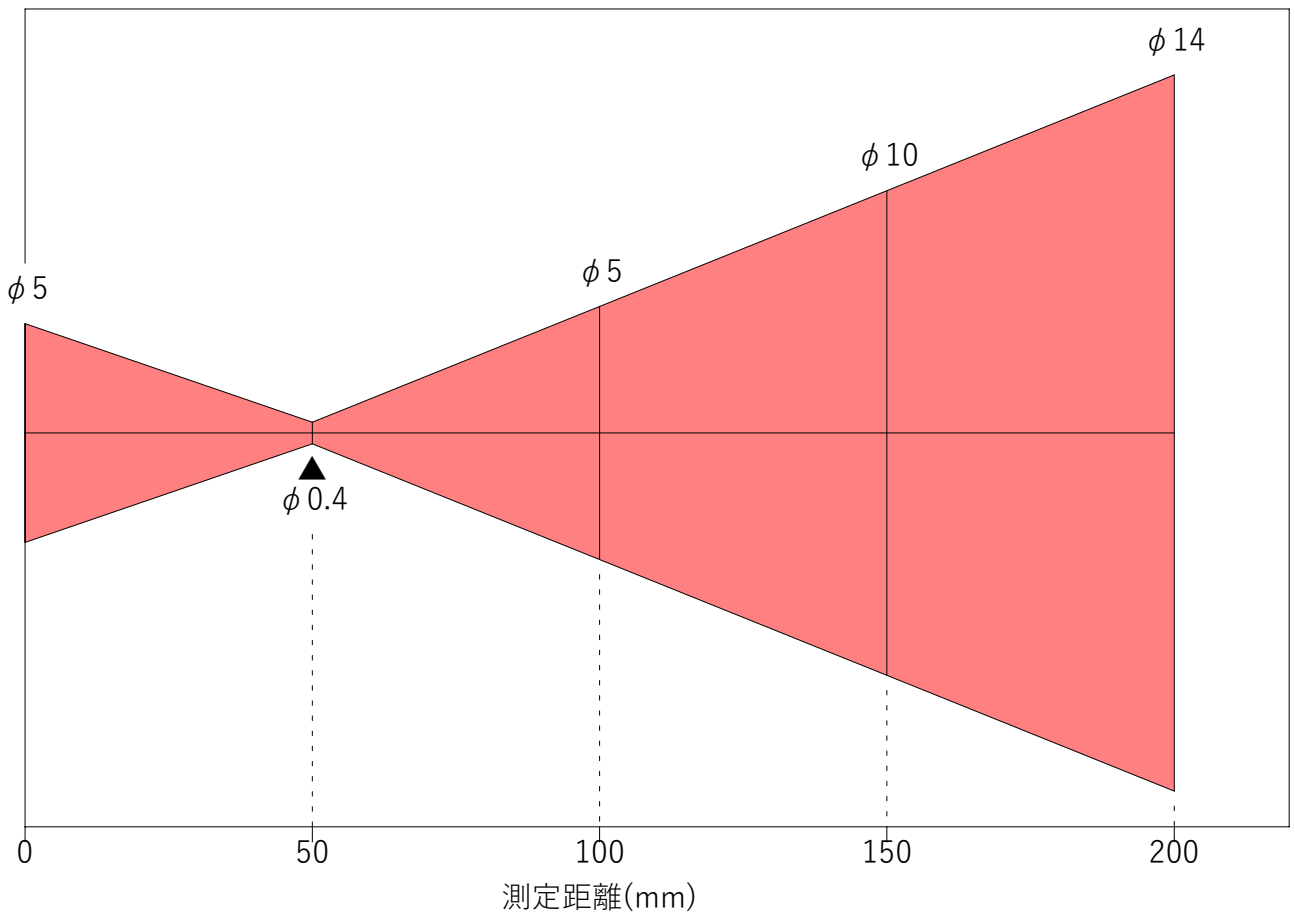
0050S1/0050R1 光路図
