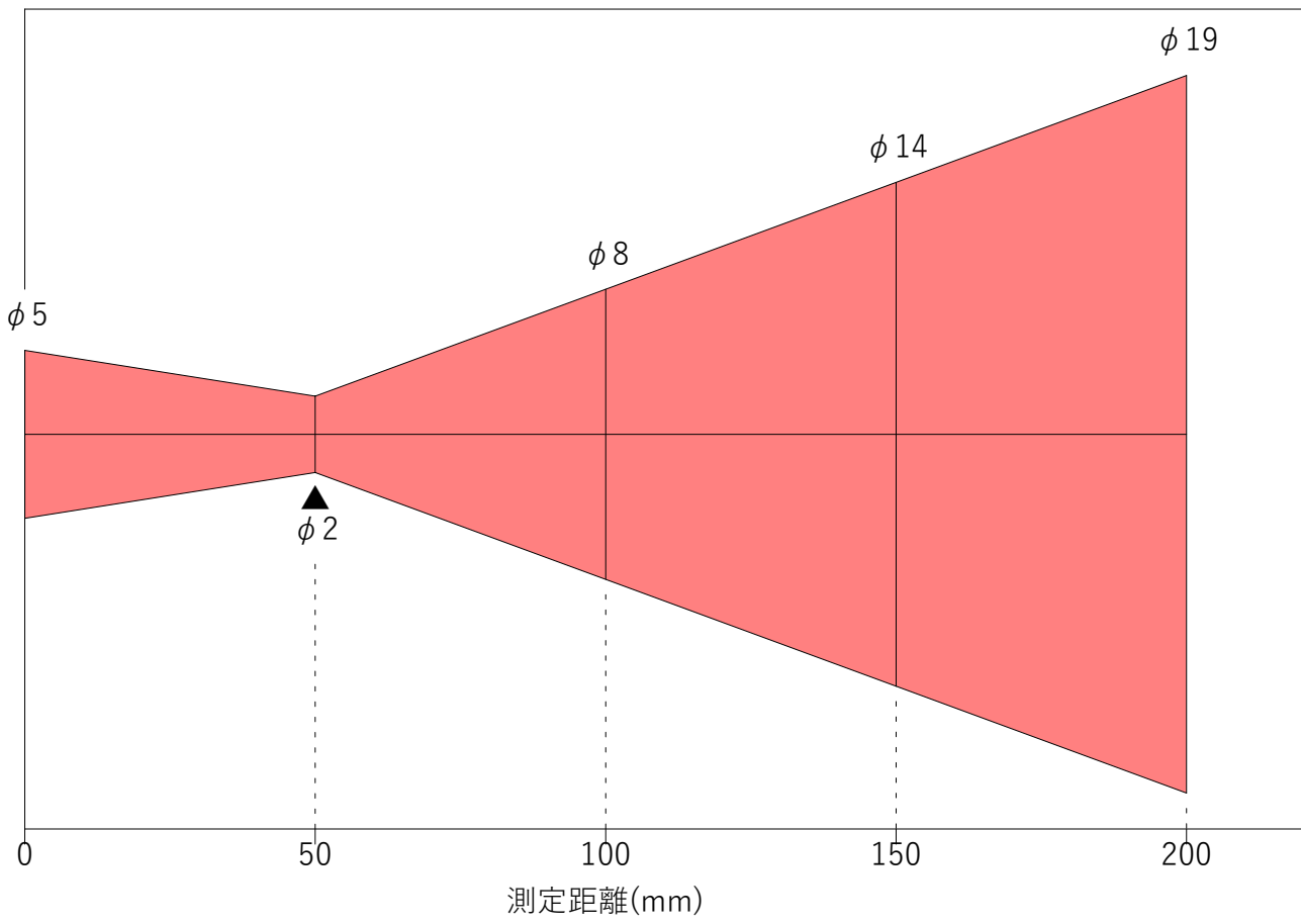
0050S002 光路図
