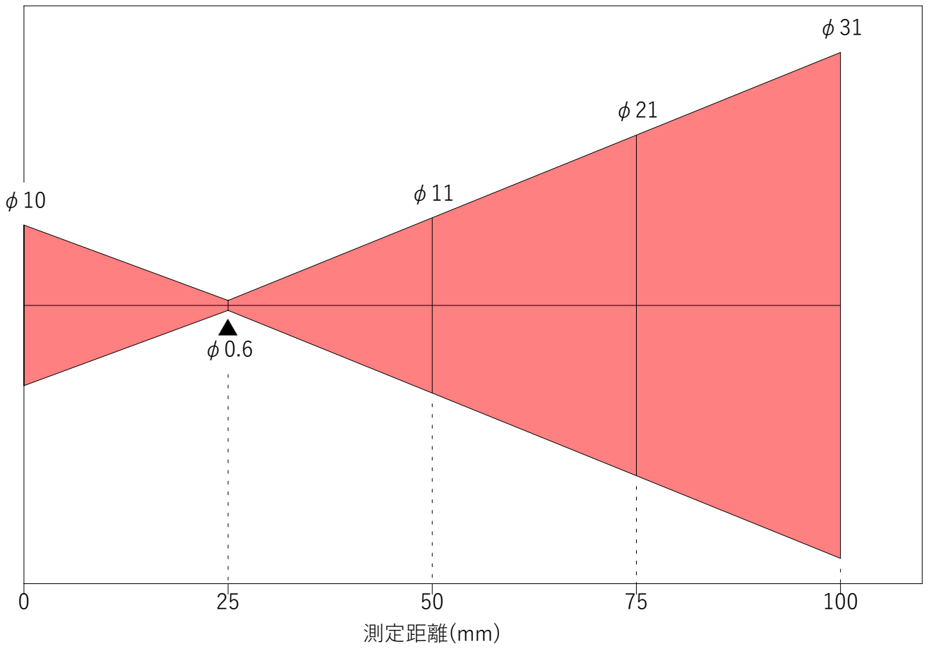
0025B6 光路図
