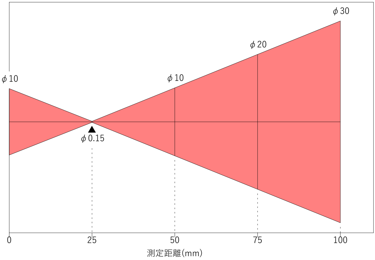
0025B1 光路図
