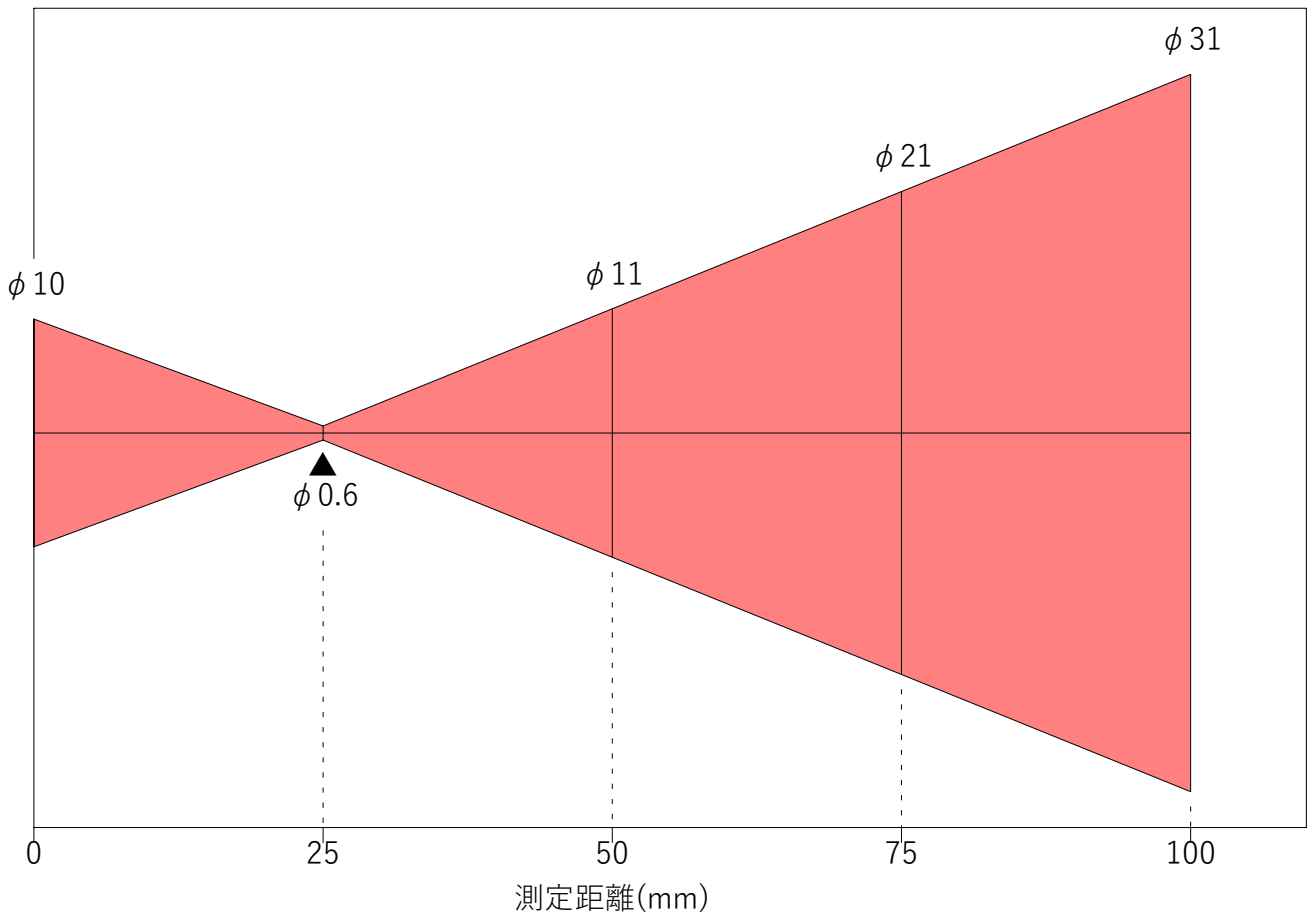
0025B0.6 光路図
