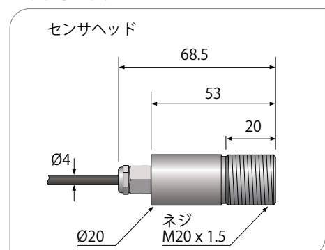
外形寸法図
