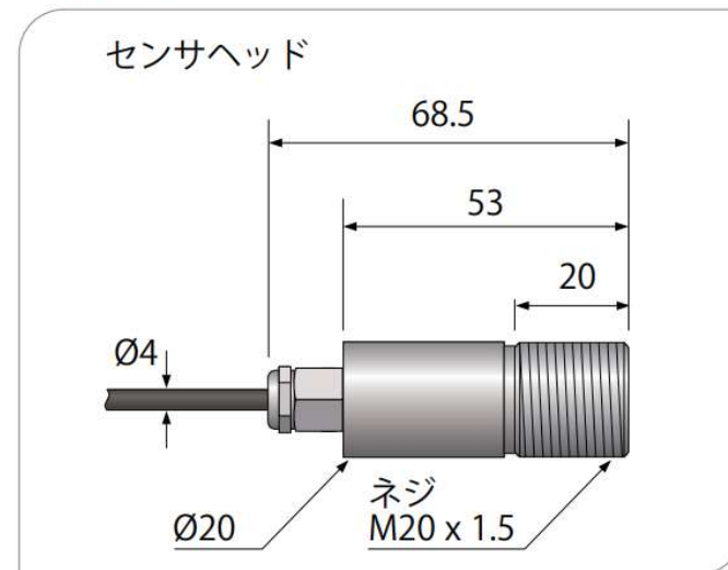
外形寸法図
