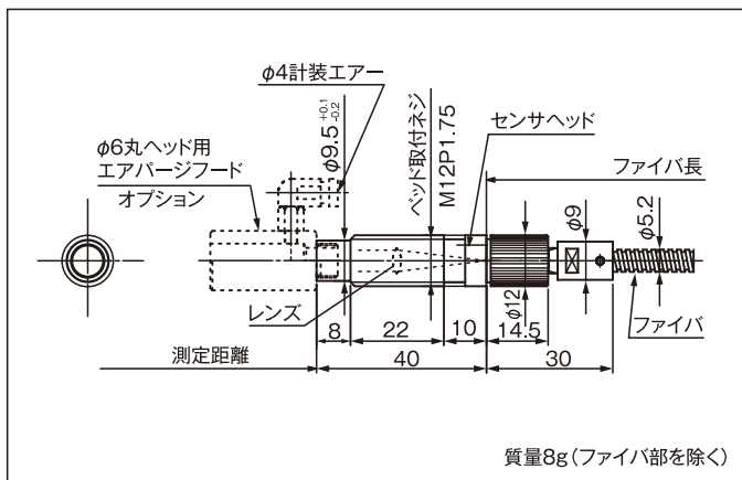
R型 Φ6レンズ 丸型ヘッド
