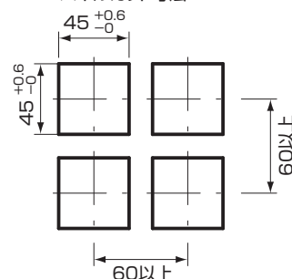
パネルカット寸法
