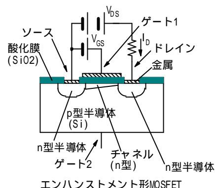
エンハンスメント形MOSFET
