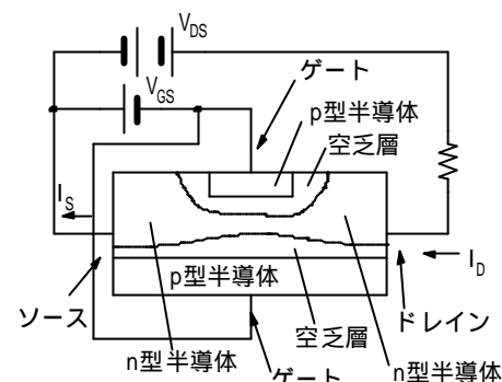
接合型FET
