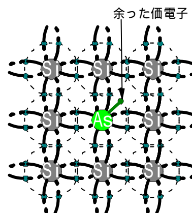
Asの元素が混入された結晶
