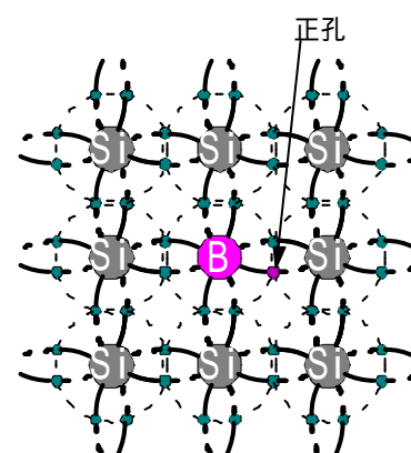
Bの元素が混入された結晶
