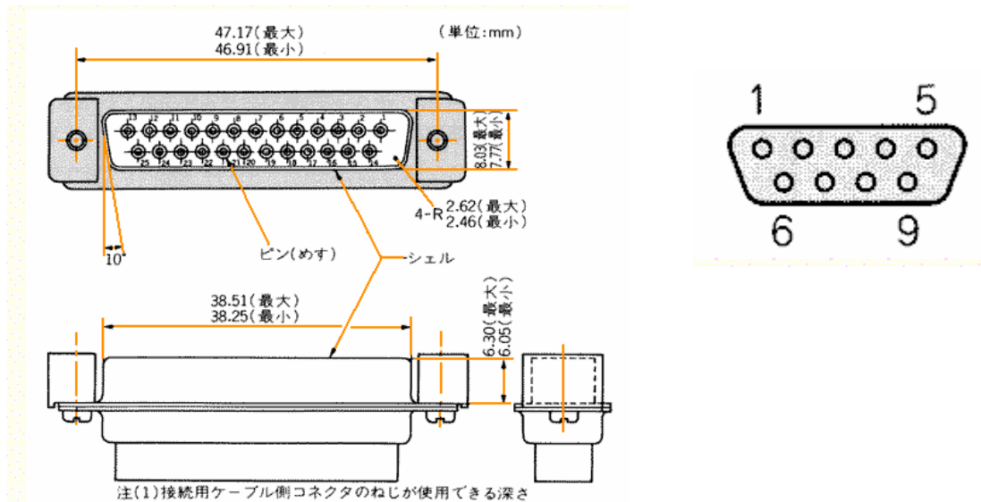
D-sub 25 ピン
