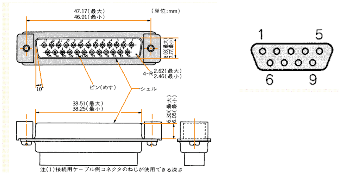
D-sub 25 ピン
